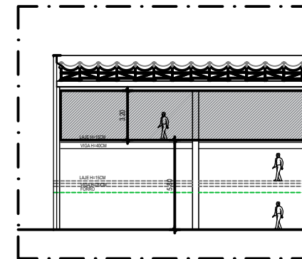
CORTE ESQUEMÁTICO ESCALA 1/200
