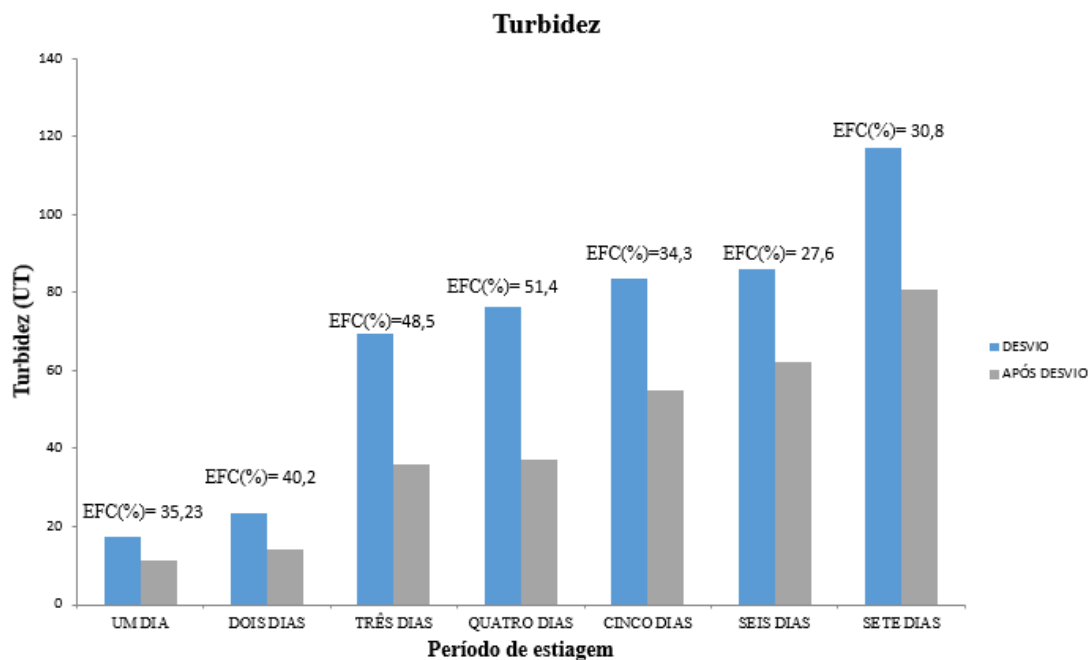
Figura 23: Média dos valores de Turbidez
