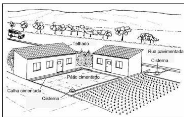
Figura 4: Projeto de captação de água de chuva denominado “1-2-1”
