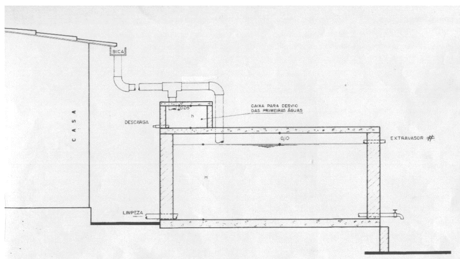
Figura 6: Dispositivo para desvio automático das primeiras águas baseado no princípio de fecho hídrico.
