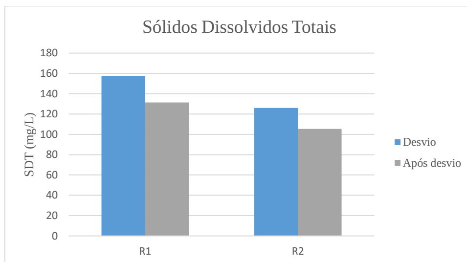
Figura 19: Média sólidos dissolvidos totais das águas de chuva armazenada na zona rural.
