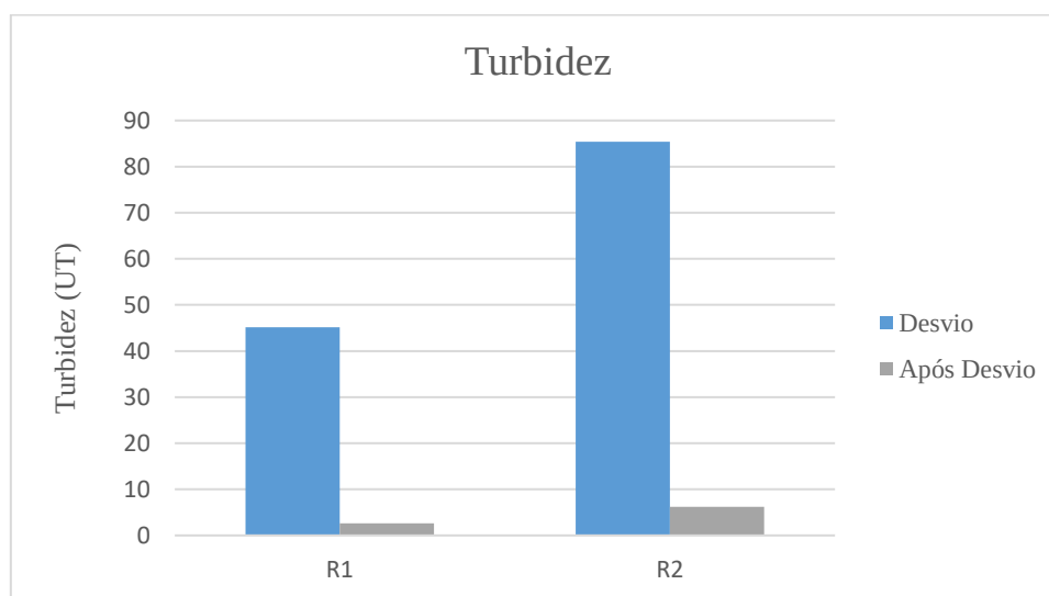
Figura 18: Média de turbidez das águas de chuva armazenada na zona rural.
