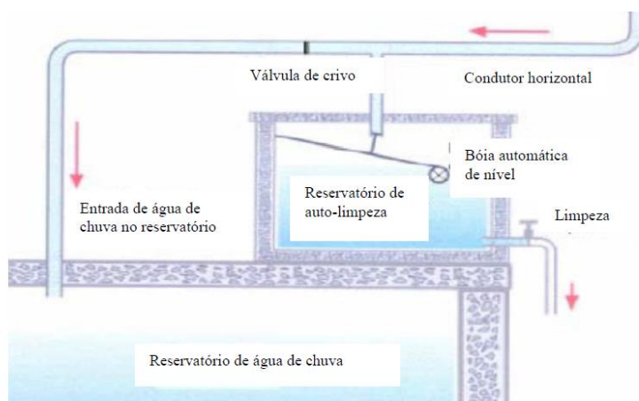
Figura 5: Esquema de cisterna com boia de nível.
