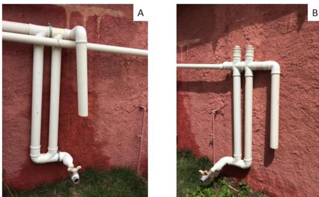
Figura 24: A-DesviUFPE na sua configuração original. B-DesviUFPE após mudança na sua configuração.
