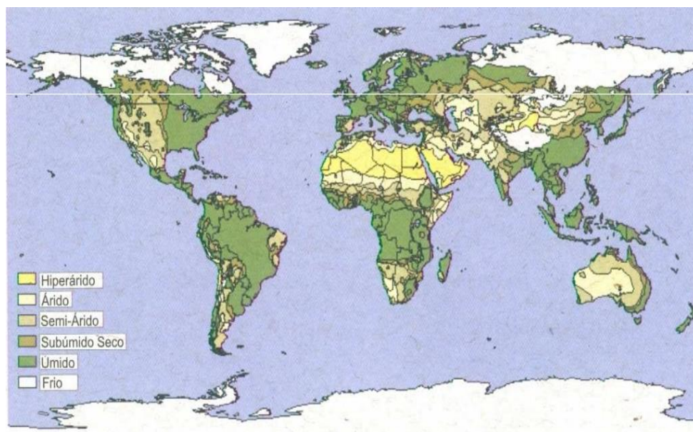
Figura 1: Climas do mundo segundo o índice de aridez
